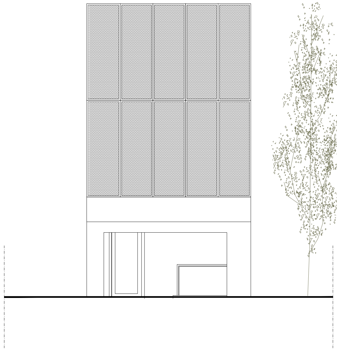
JUŽNO PROČELJE MJ 1:100
